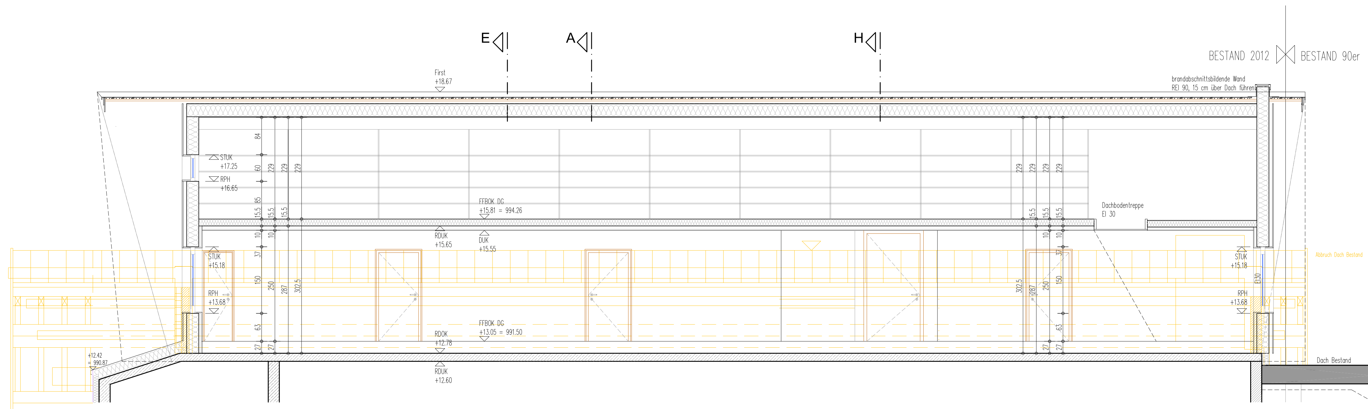
Schnitt B
