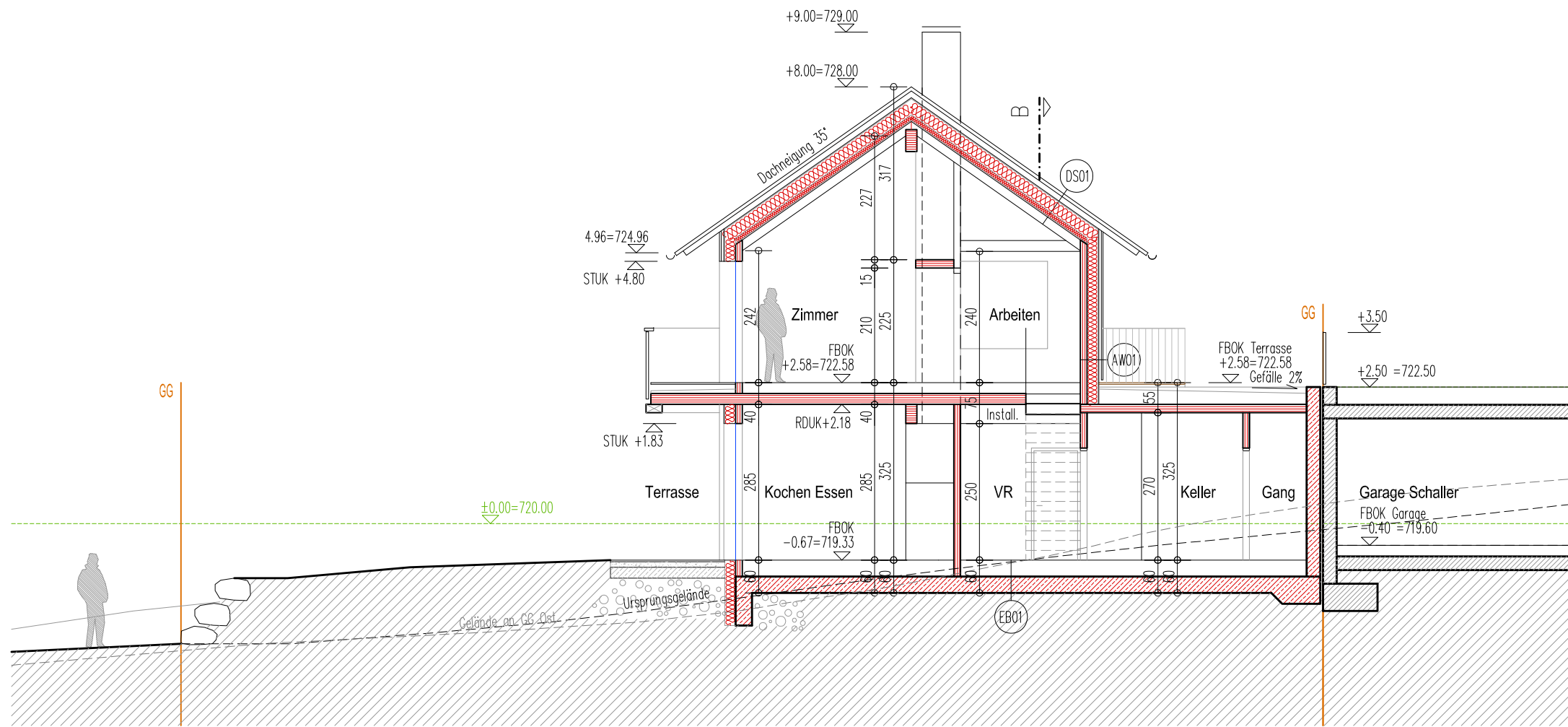
Schnitt A-A
