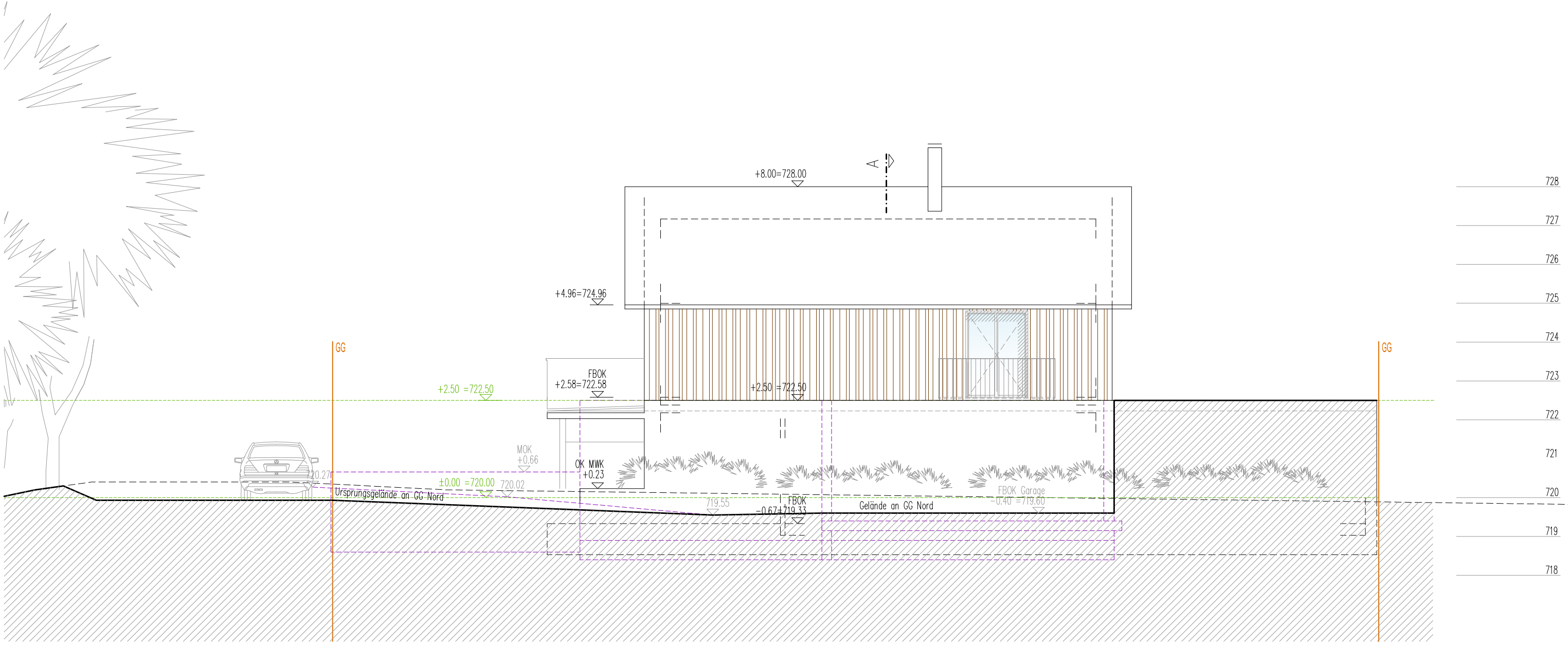
Ansicht Nord
