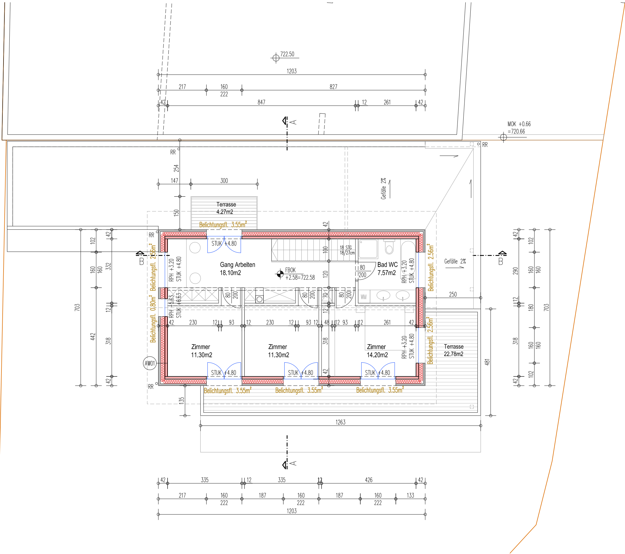
Grundriss Obergeschoss
