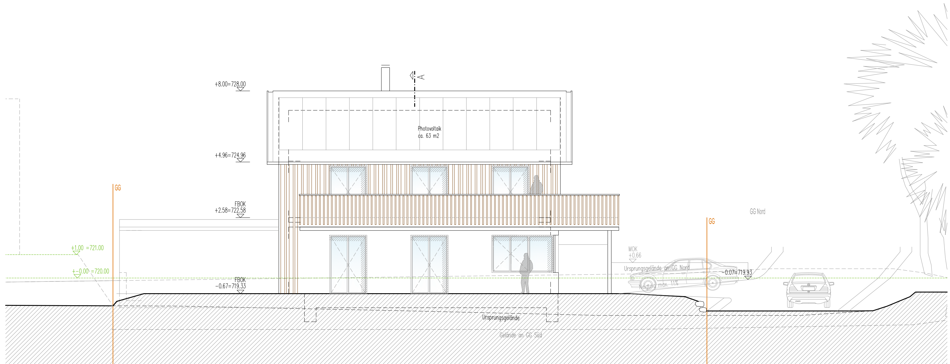
Ansicht Süd
