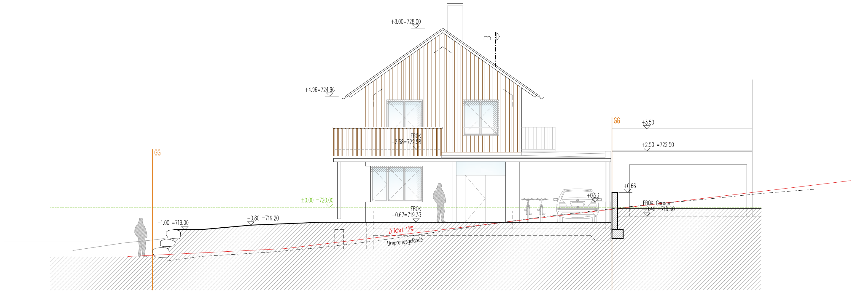
Ansicht Ost
