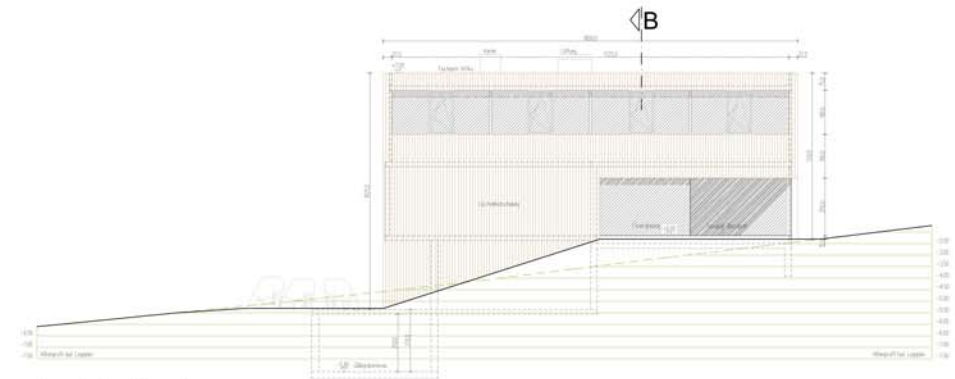
Ansicht Nord
