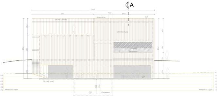
Ansicht Ost
