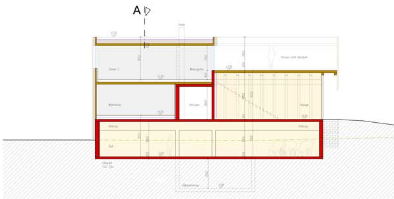
Schnitte B-B
